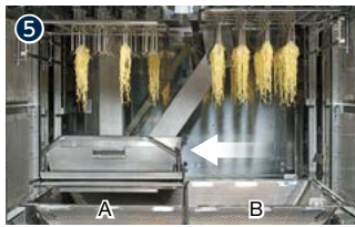
⑤ 把持部Bのハンドでマッチング計量し、バットが把持部Aへ移動
