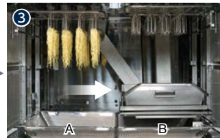
③ 把持部Aのハンドでマッチング計量し、バットが把持部Bへ移動
