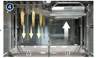
④ 把持部Aでマッチング計量された商品を排出 バットが上昇、把持部Bのハンドで商品を掴む
