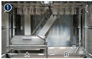
① 商品が充填されたバットを装置内(把持部A)へセット
