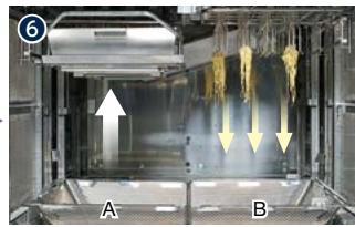
⑥ 把持部Bでマッチング計量された商品を排出 バットが上昇、把持部Aのハンドで商品を掴む
