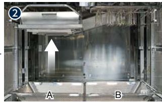
② バットが上昇、把持部Aのハンドで商品を掴む
